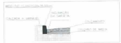
DETALHE DA SARIETA SEM ESCALA
